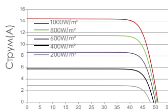
Напряга (В)
