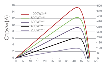
Напряга (В)
