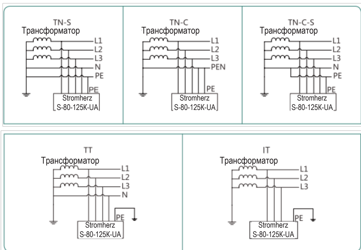
Малюнок 3-1 Застосовні типи мережі для інвертора з виходом 400В
