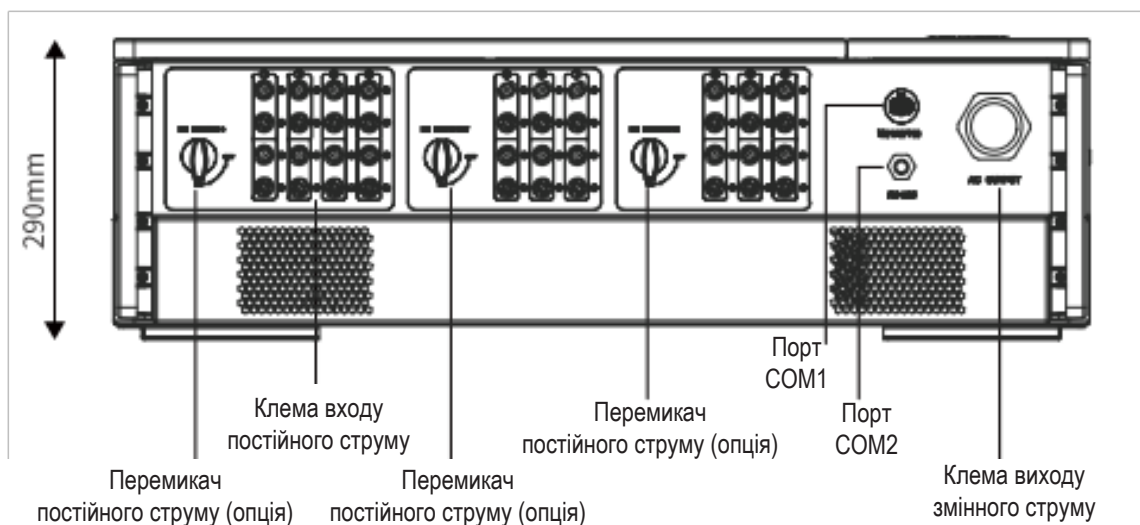
Малюнок 3-5 Вигляд знизу
